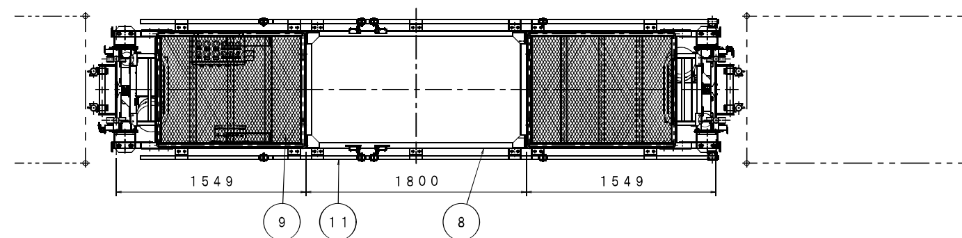
平面図 (S=1:30)
