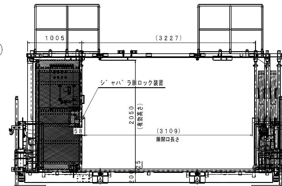
扉開時正面図 (S=1:30)
